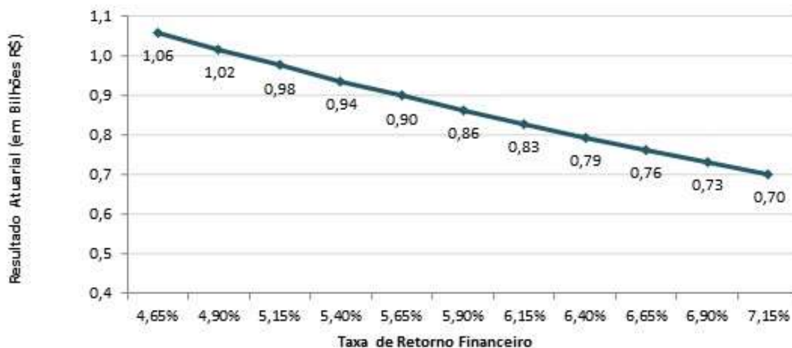
Gráfico 9: Variação do Resultado Atuarial em Função da Taxa de Juros Real
