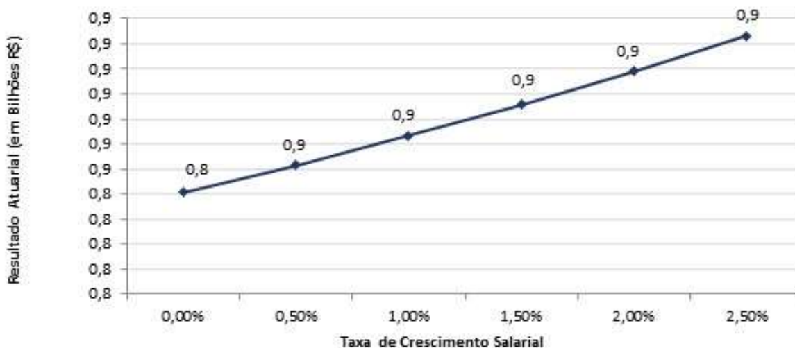
Gráfico 10: Variação do Resultado Atuarial em Função do Crescimento Salarial
